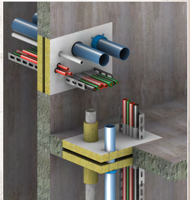
Brandabschottung
